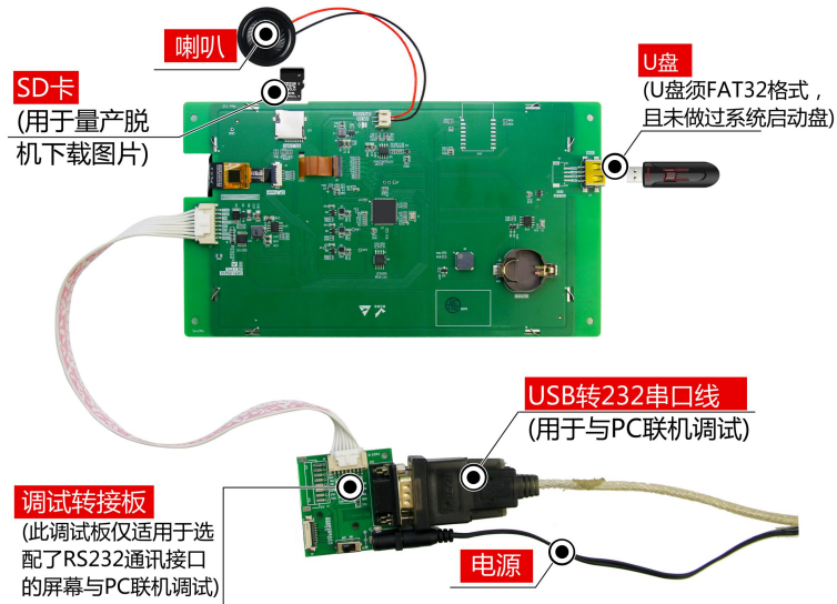
图 1-4 调试工具图
