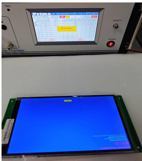
图 4-3 EFT 测试图
