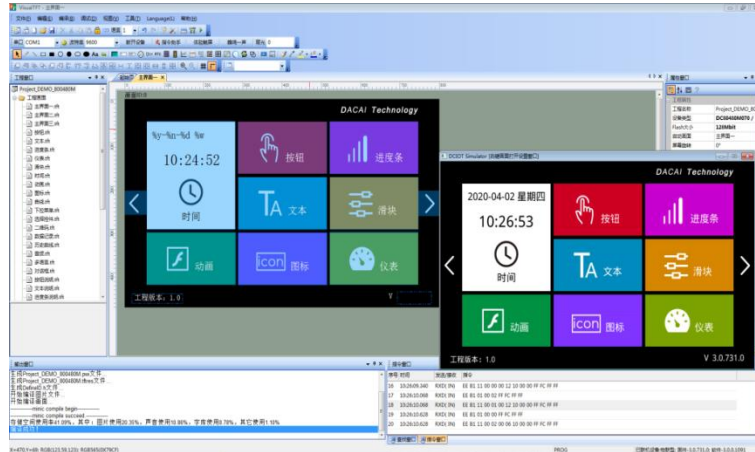
图 6-1 VisualTFT 主界面
